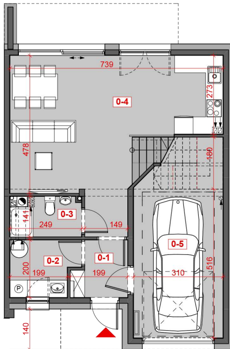
POGLĄDOWY RZUT PARTERU
