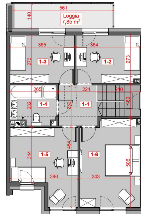
POGLĄDOWY RZUT PIĘTRA
